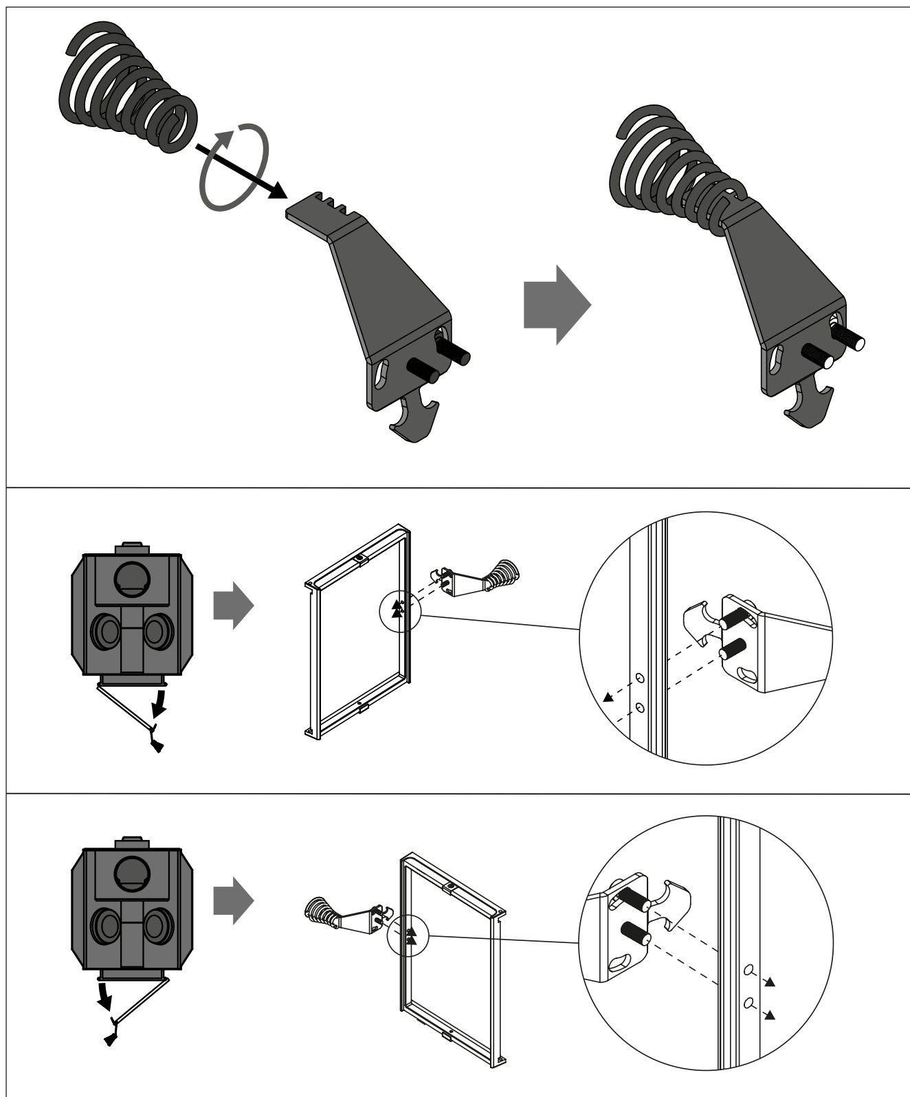
Рисунок 13. Изменение стороны подвески дверцы каменки
