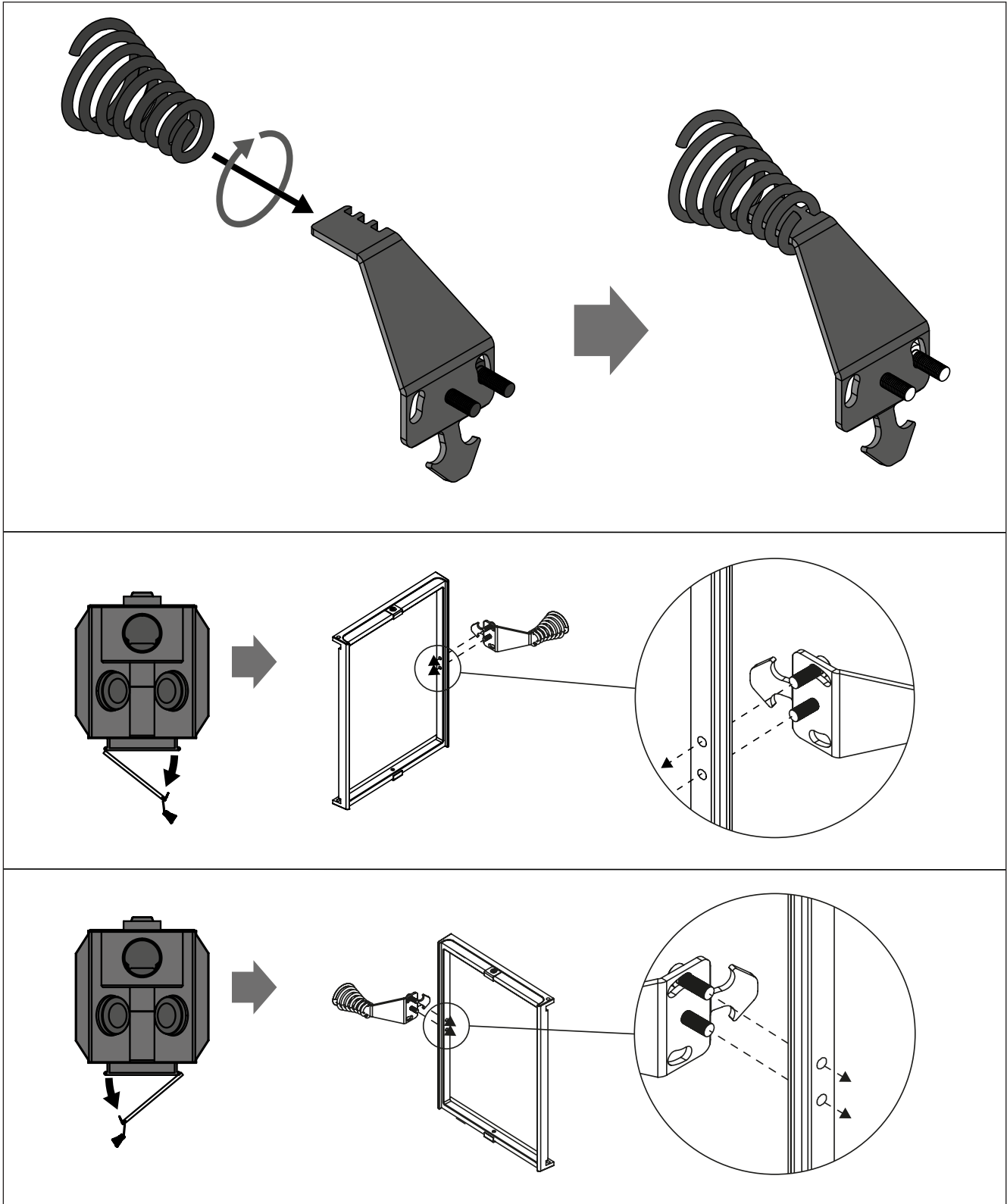
Kuva 13. Luukun käsisyyden vaihtaminen Bild 13. Byte av luckans öppningsriktning
