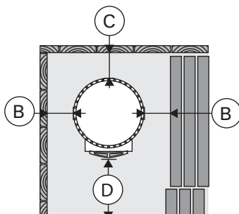
Рисунок 9. Безопасные расстояния (все размеры приведены в миллиметрах)
