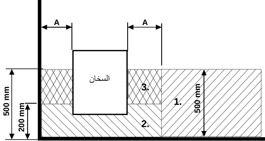
صورة 3 وضع صندوق التوصيلات بكبل التوصيل في غرفة الساونا
