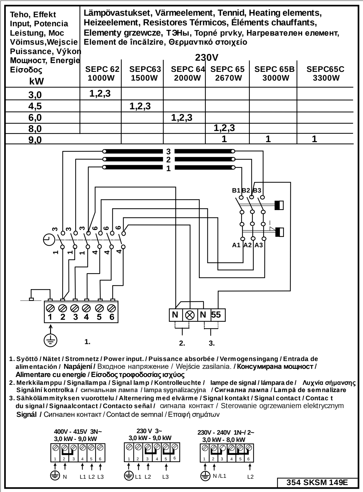
Imagen 4 Diagrama de conexiones
