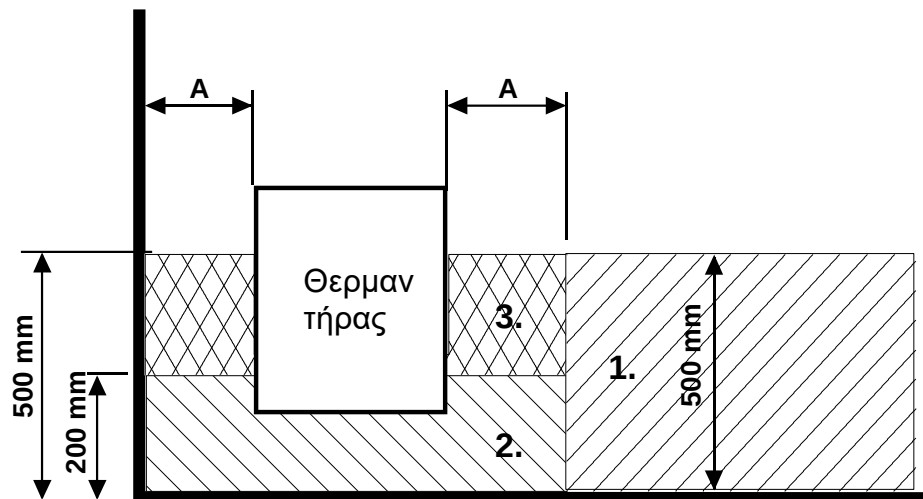
Εικόνα 3 Θέση του κυτίου σύνδεσης για το καλώδιο σύνδεσης στην αίθουσα σάουνας
