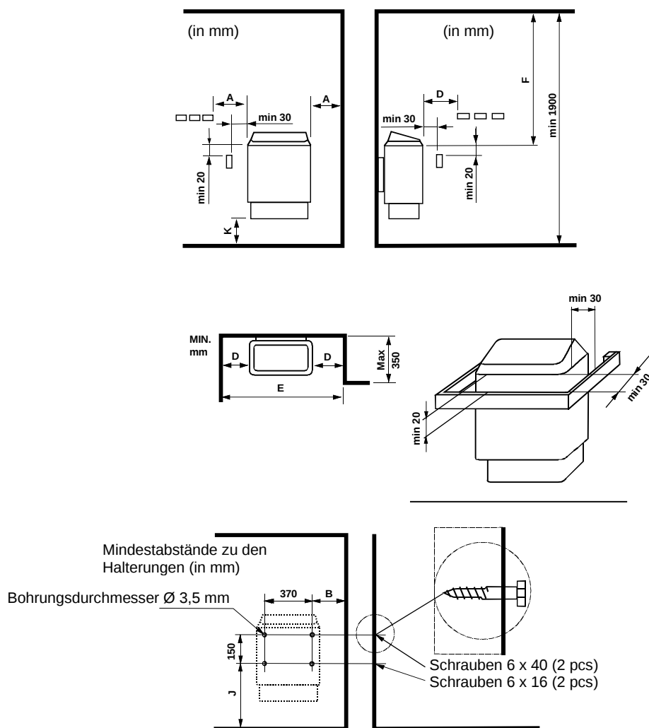
Abbildung 2 Sicherheitsabstände
