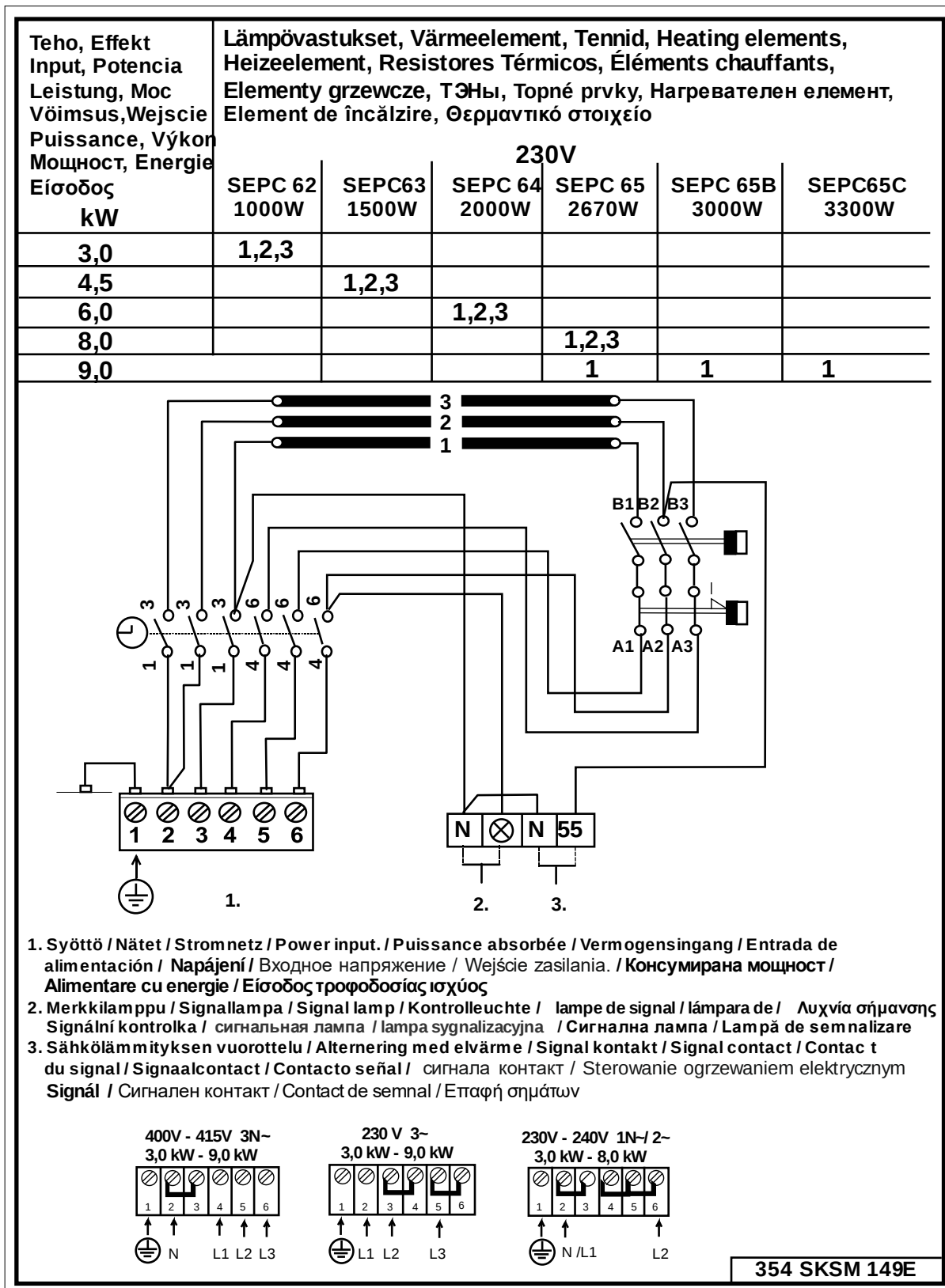
Bild 4 Kopplingsschema
