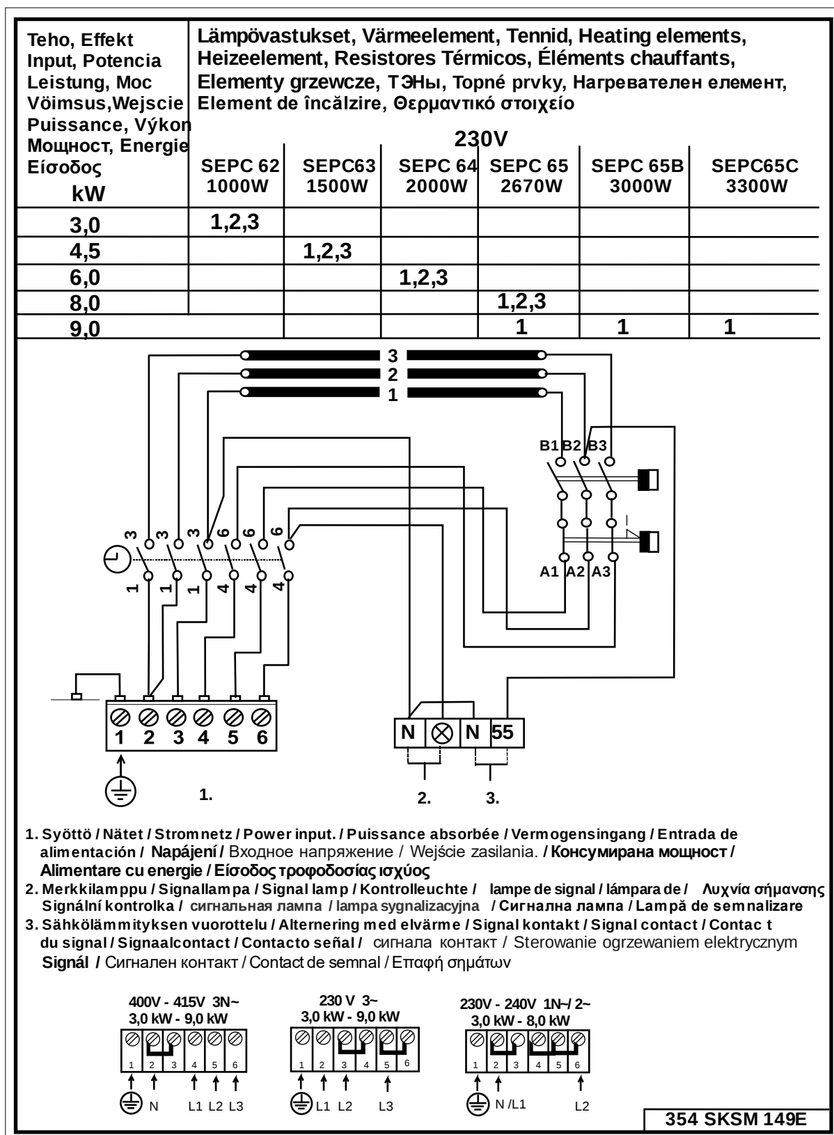
Рис. 4 Схема электрических соединений
