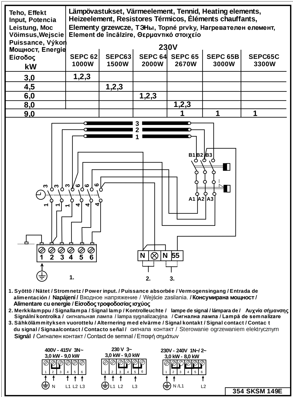
Kuva 4 Kytentäkaava
