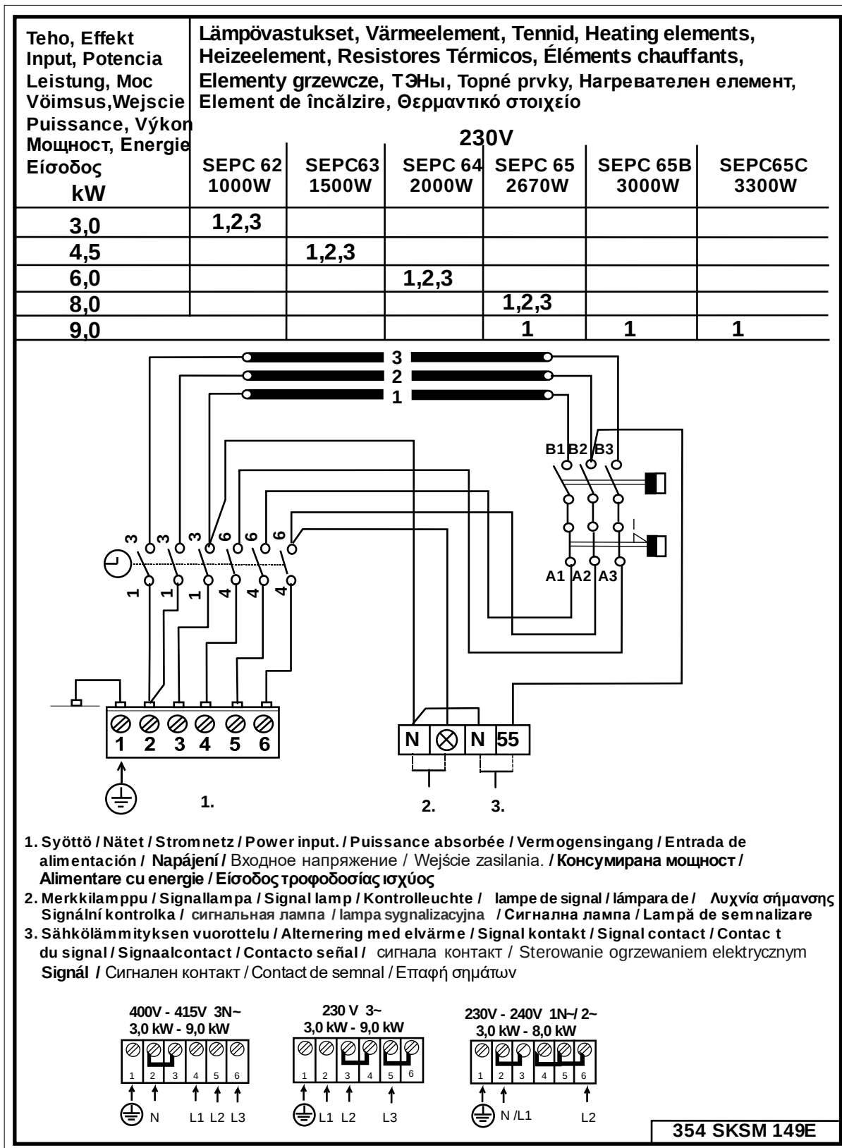
Obrázek 4 Schéma zapojení
